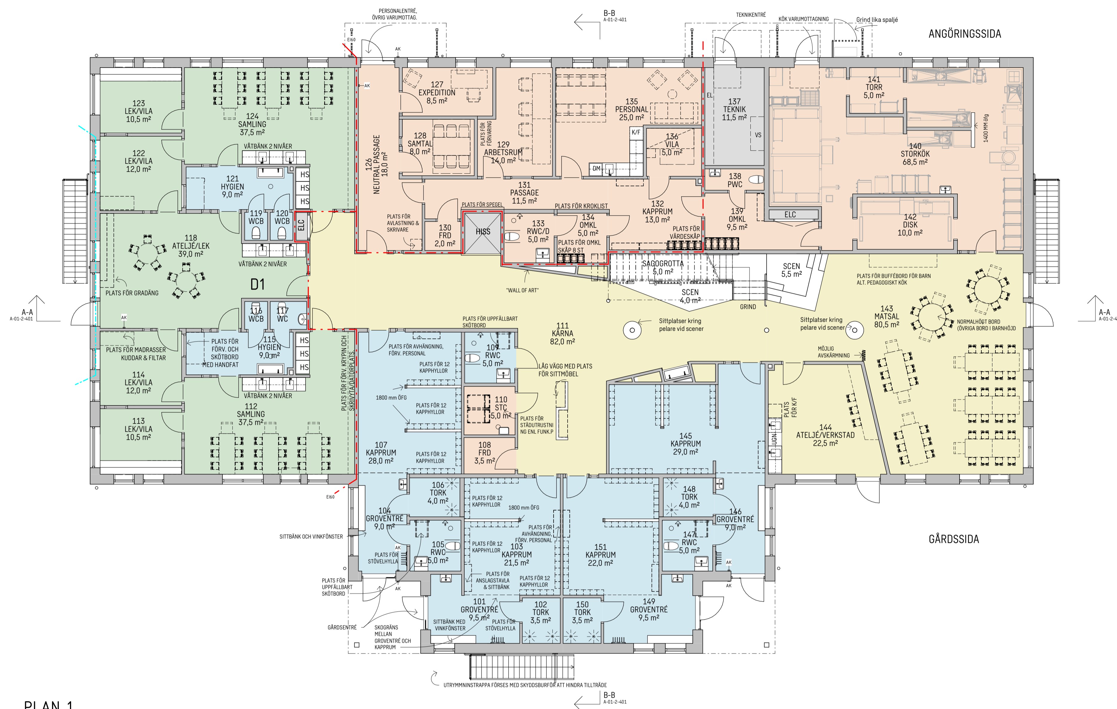
PLAN 1 1 : 100
